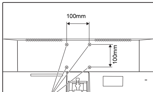
アーム、壁掛けキット固定用ネジ穴
